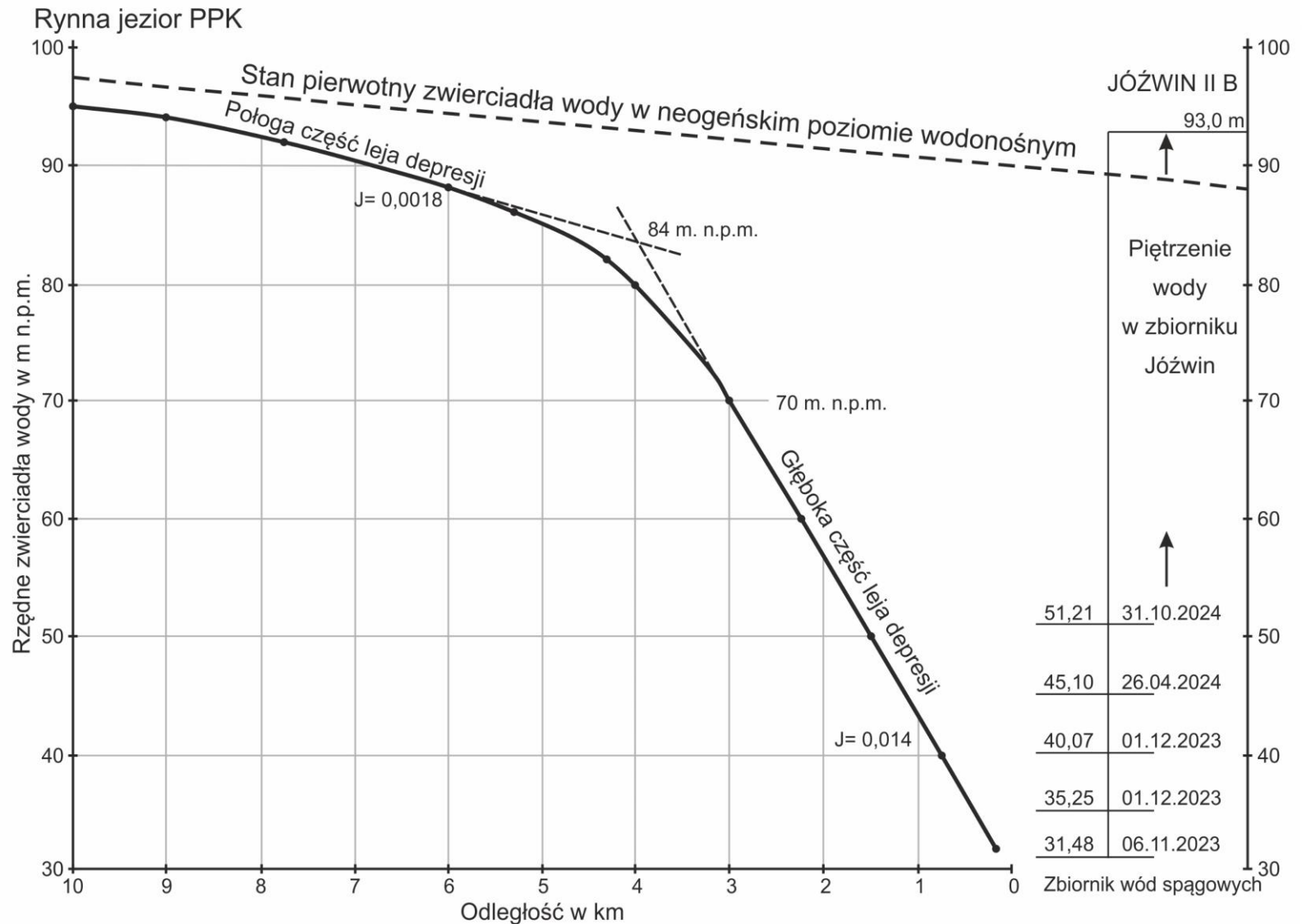
Rys. 1. Profil leja depresji o/Józwin II B i wypełnianie się wodą podziemną zbiornika powyrobiskowego
