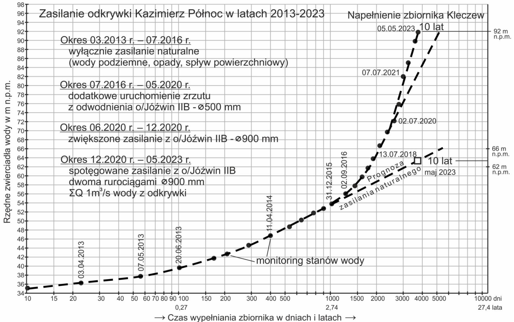
Rys. 4. Przyrost zwierciadła wody w funkcji s=f(\lg t) na podstawie pomiarów i prognozy hydrogeologicznej
